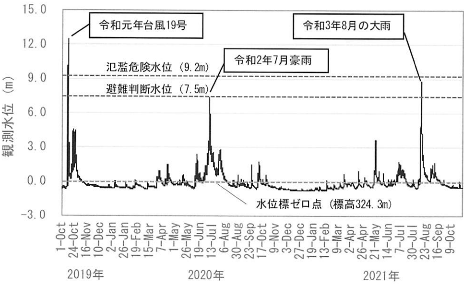
図2 2019年10月から2021年10月までの立ヶ花観測所の観測水位 (立ヶ花観測所の観測水位データより)
