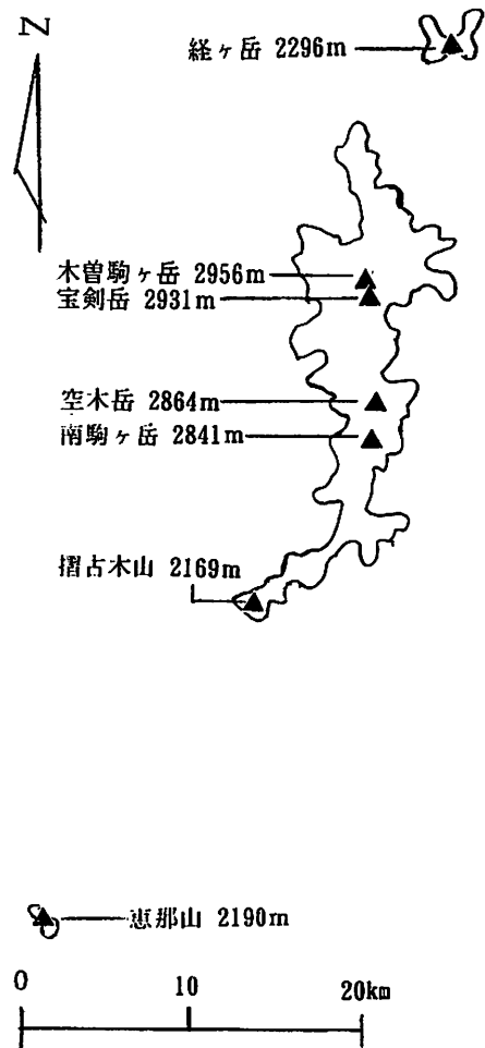
中央アルプスの山岳名と標高 (等高線は、標高2000m)
