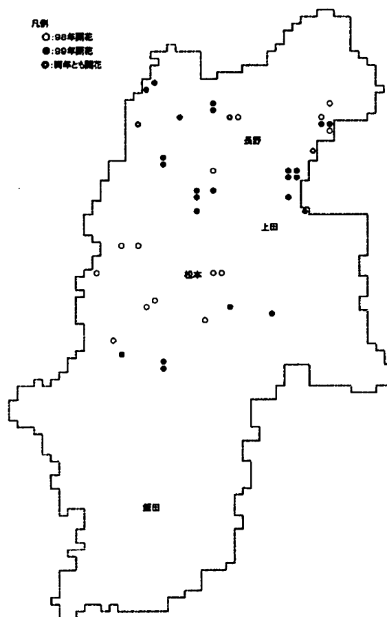
図-1 長野県内のササ開花記録位置図(1998年および1999年)
